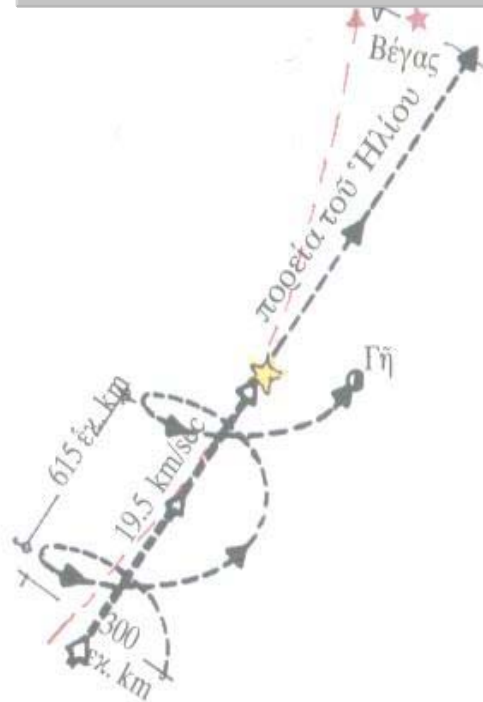
Σχ. 7. Η κίνηση του Ήλιου και η έλικοειδής κίνηση της Γης.
